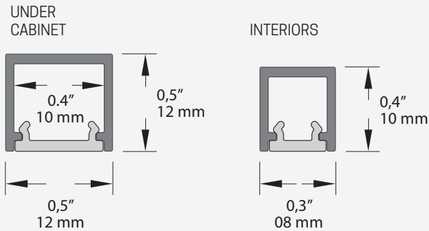
Profile section Sezione canalina
