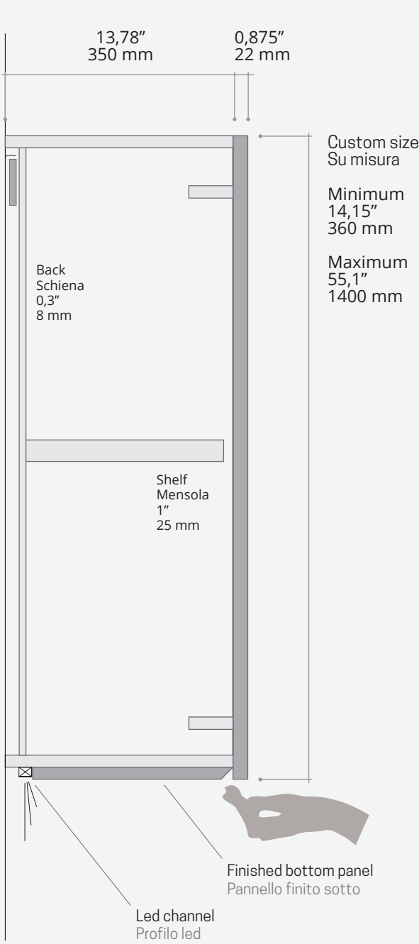
Upper cabinet side section Pensili sezione laterale
