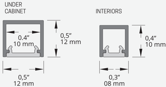
Profile section Sezione canalina
