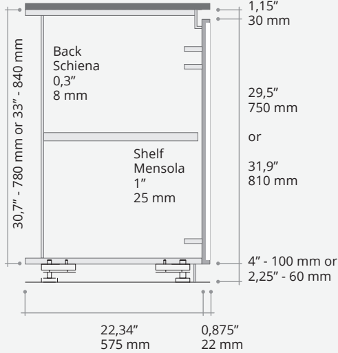
Base cabinet side section Sezione laterale basi
