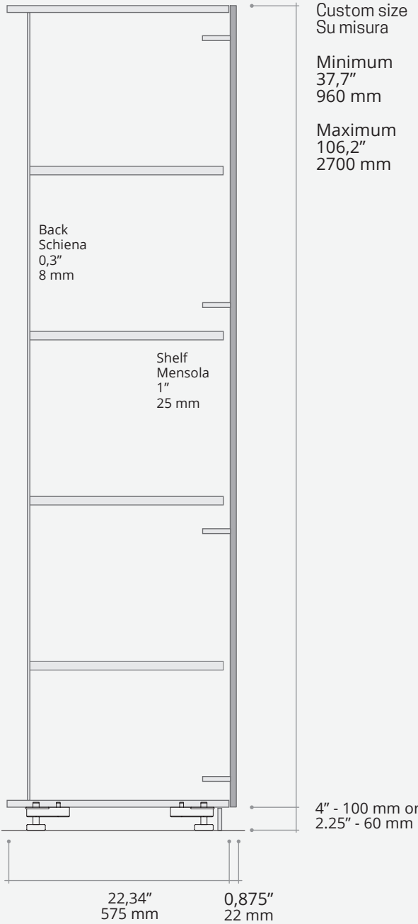
Column side section Colonna sezione laterale
